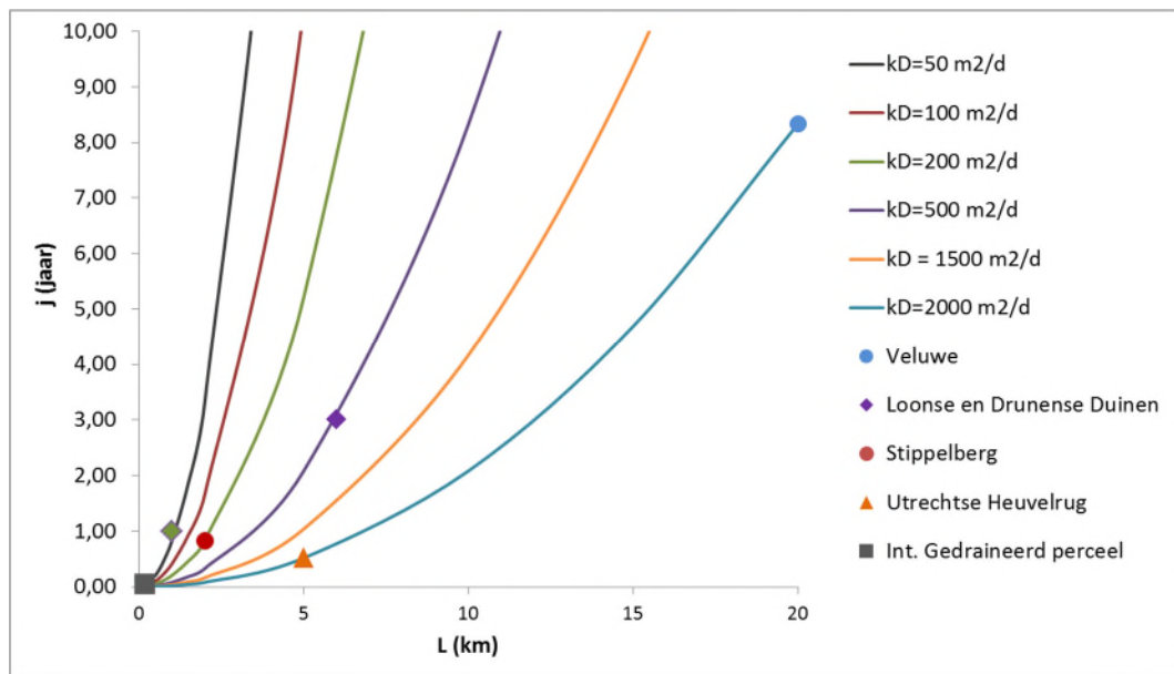
Figuur IV-1: Reservoircoëfficiënt als functie van de afstand tussen drainerende elementen voor een aantal doorlaatvermogens ( kD , m^2/d ) berkend op basis van Kraijenhoff van de Leur (1958)
